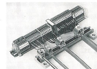
Woertz-Schirmanschlussklemmen
