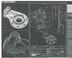
Anwendungsbeispiele von CAD/ CAM-Software
