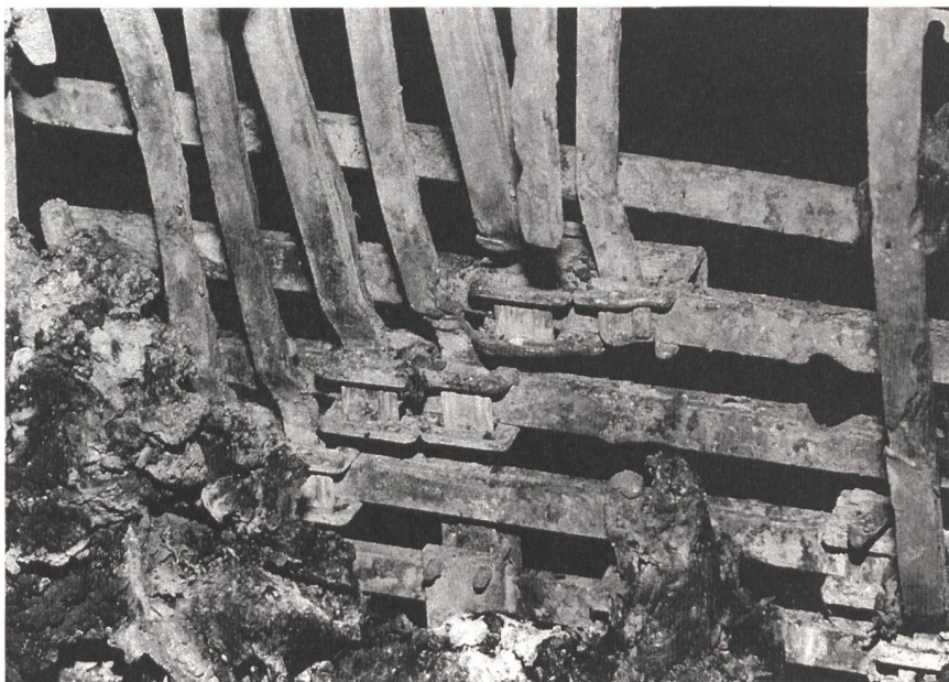
Bild 1 Ein durch Überlast zerstörter Niederspannungsverteiler
