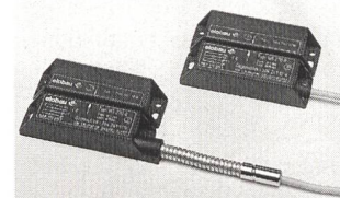
Sicherheitsschalter und Betätigungsmagnetsystem
