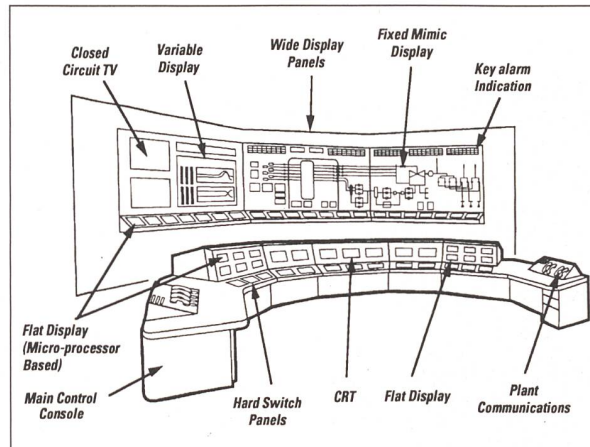
Caractéristiques du centre de contrôle du réacteur à eau bouillante (ABWR/GE).
