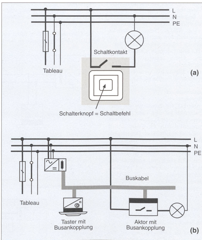
Bild 9 Vergleich zwischen traditioneller Installation und Bussystem
