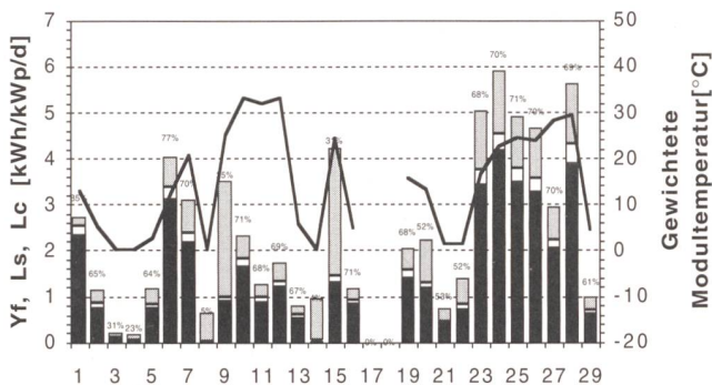
Bild 10 Kenngrossen (Tagesmittelwerte) der PV-Anlage Neu-Technikum Buchs im Monat Februar 1996.
