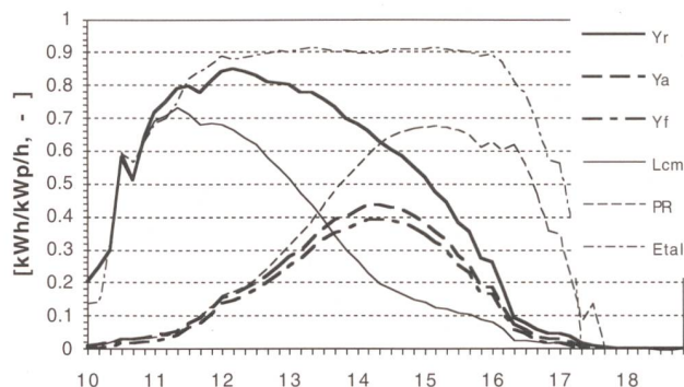
Bild 11 Tagesverlauf der wichtigsten Kenngrossen der Photovoltaikanlage am NTB am Beispiel des 15. Februars 1996.
