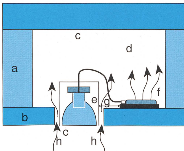
Figure 1 Schéma de montage.
