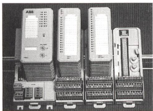
Advant Controller 70 mit zwei Ein-/Ausgangsmodulen und einer freien Anschlusseinheit
