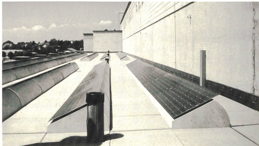
Bild 1 Solare Pilotanlage mit Betonsockeln als Tragkonstruktion (Solarmodule auf dem Dach der ETH Lausanne VD). (Fotos: EPFL/PMS/Enecolo AG)
