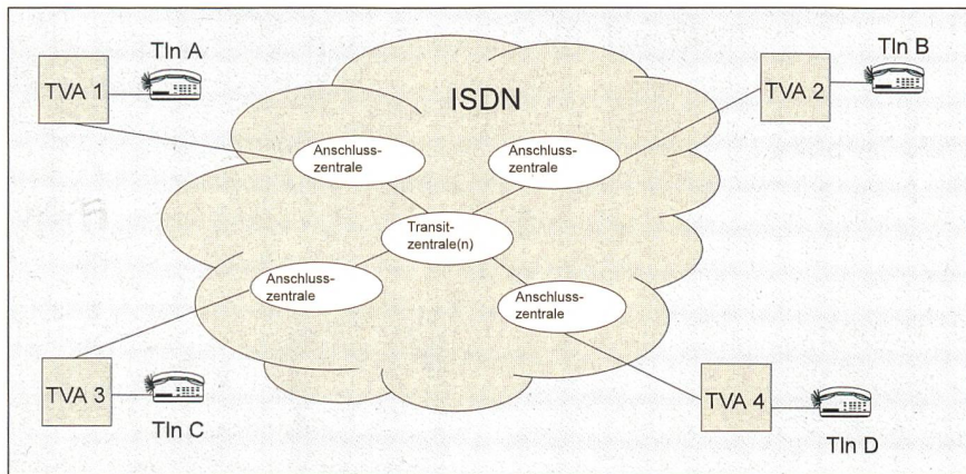
Bild 2 Virtuelle Vernetzung
