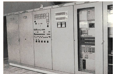
Bild 4 Die neue Bedientafel in der Zentrale Safien. Bei Unterhaltsarbeiten und in Ausnahmesituationen wird die Schaltanlage von hier aus bedient. Im Normalbetrieb erfolgt die Bedienung der Zentrale Safien von der zentralen Leitstelle in Rothenbrunnen aus.
