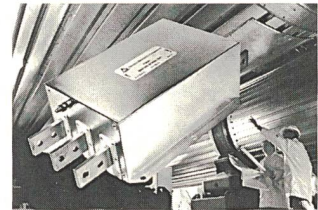
Rauhe Burschen: EMV-Filter bis 2500 A
