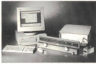
PAMP 250 für RF-Prüfung gemäss IEC 1000-4-6
