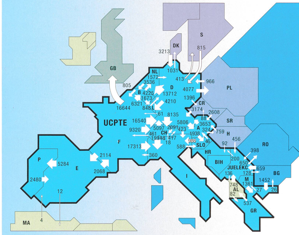
Stromtausch 1997 im europäischen Verbundsystem (physikalische Energieflüsse in GWh; Quelle UCPTÉ)
