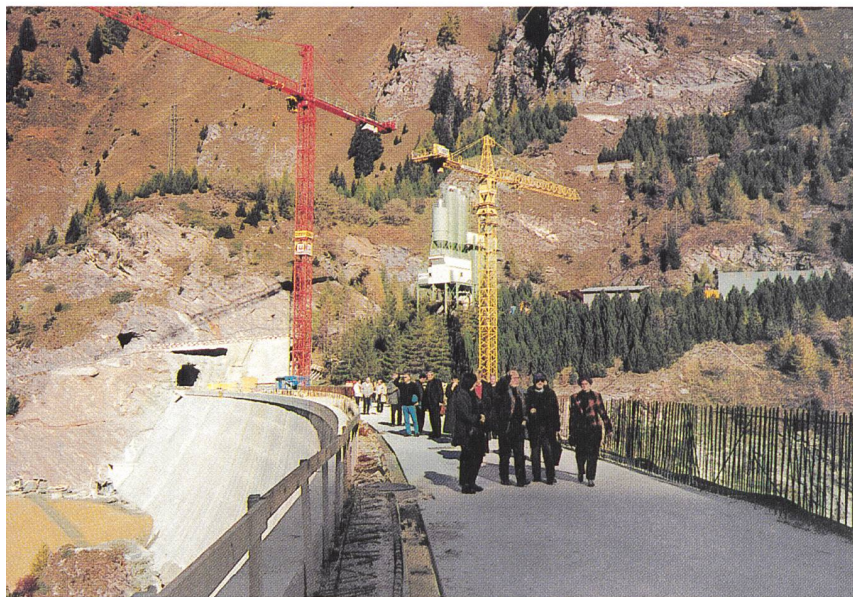
Erste Besichtigungen auf der um 17 Meter erhöhten Staumauer von Luzzzone (TI).
