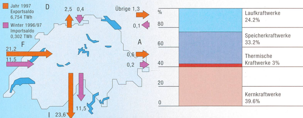
Anteil der Kraftwerktypen an der Schweizer Stromproduktion 1997
