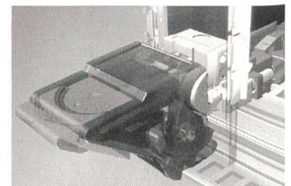
Ergonomischer Griff für hochpolige Steckverbinder
