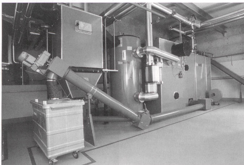
Bild 1 Holzschrottel-Rostfeuerung von Tiba-Müller AG mit 3 MW Wärmeleistung.
