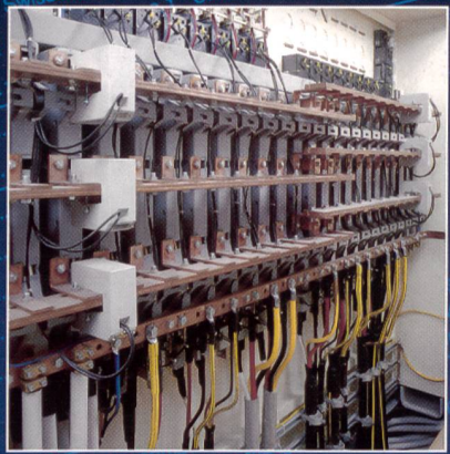
Schienensystem: flachliegend/horizontal
