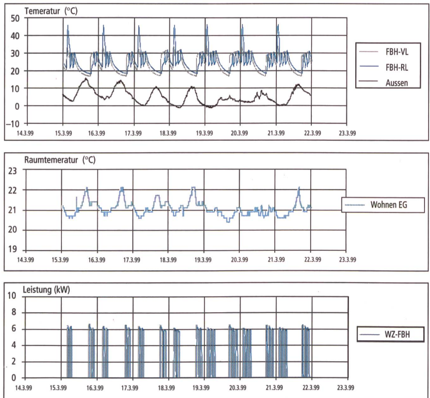
Bild 1 Messergebnisse für die Woche 99-11 als Beispiel. FBH-VL: Vorlauf temperatur der Fussbodenheizung, FBH-RL: Rücklauf temperatur der Fussbodenheizung, Aussen: Aussentemperatur, WZ-FBH: Wärmemähler Fussbodenheizung (aus Schlussbericht).
