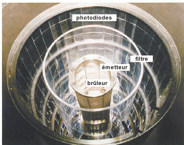
Fig. 5 Intégration d'un système TPV dans une chaudière à gaz de 20 kW
