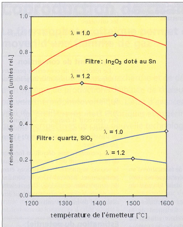
Fig. 4 Optimisation de la température de l'émetteur
