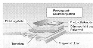
Sandwich aus Photovoltaikmodul und Polystyrol
