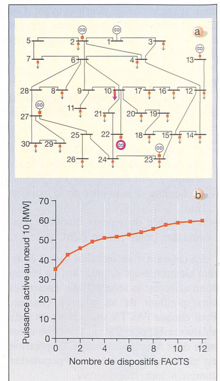
Fig. 10 Simulation d'échange entre producteur et consommateur proches: a) localisation sur le réseau; b) puissance active échangeable entre ces deux nœuds en fonction du nombre de FACTS
