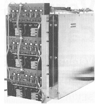
COS- \phi -Kompensationsanlage von Bajog
