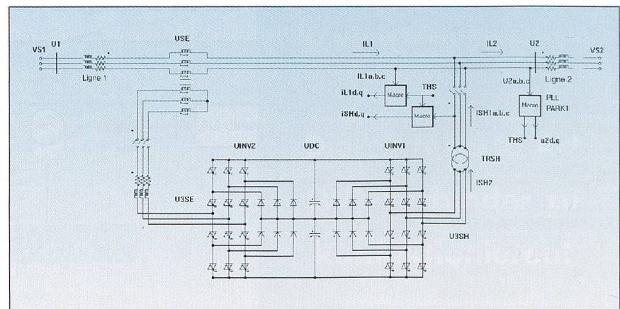
Fig. 5 Schéma de l'UPFC trois niveaux dans le simulateur Simsen
