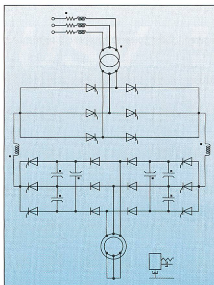
Figure 4 Schéma de l'installation
