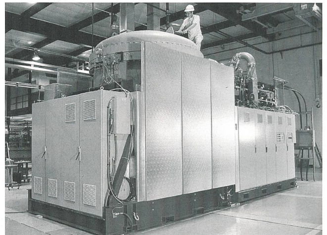
Brennstoffzellen, gekoppelt mit Gasturbine.
