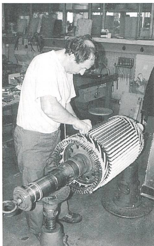
Elektromotoren-Montage (Profilwicklung).
