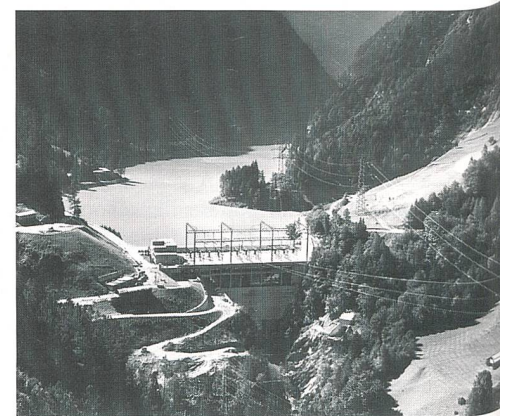
KW Sarganserland: Schwergewichtsmauer mit Zentrale und Freiluftschaltanlage des Ausgleichbeckens Mapragg (Bild: NOK).
