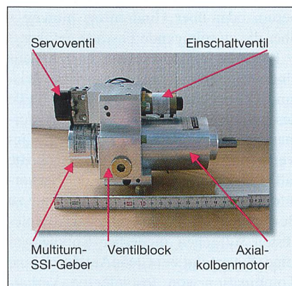
Bild 7 Axialkolbenmotor mit integriertem Ventil- und Geberblock
