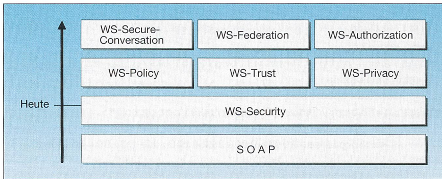
Bild 3 WS-Security
