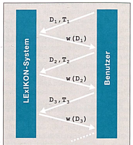
Bild 3 LEXIKON-Lern-Dialog
