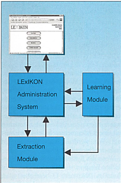
Bild 4 LEXIKON-Architektur
