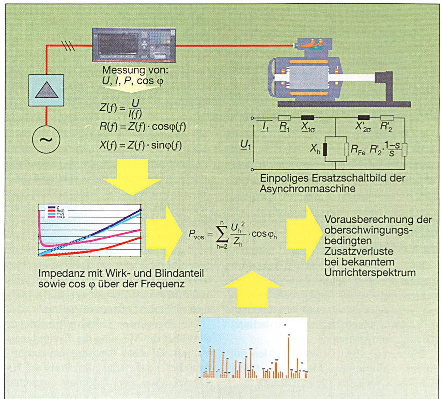
Bild 7 Ablaufschema zur Vorausberechnung der Oberschwingungsverluste
