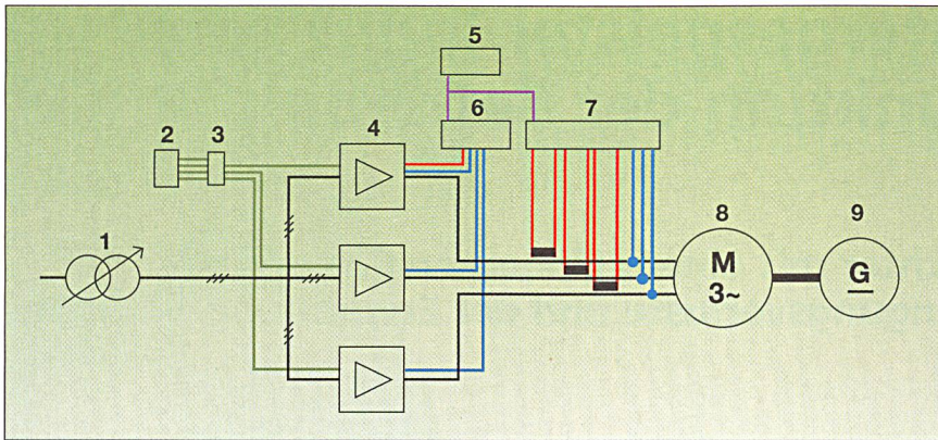
Bild 2 Schaltbild Versuchsaufbau
