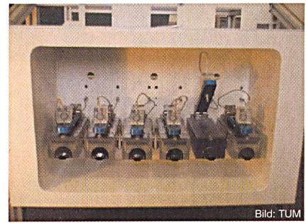
Bild 5 Frontalansicht eines 6-Kanal-Mikrophysiometers
