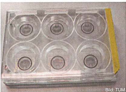
Bild 4 Eine weitere Entwicklungsrichtung ist die Konstruktion von Multititerplatten, deren Böden durch multiparametrische Sensorchips ersetzt werden.
