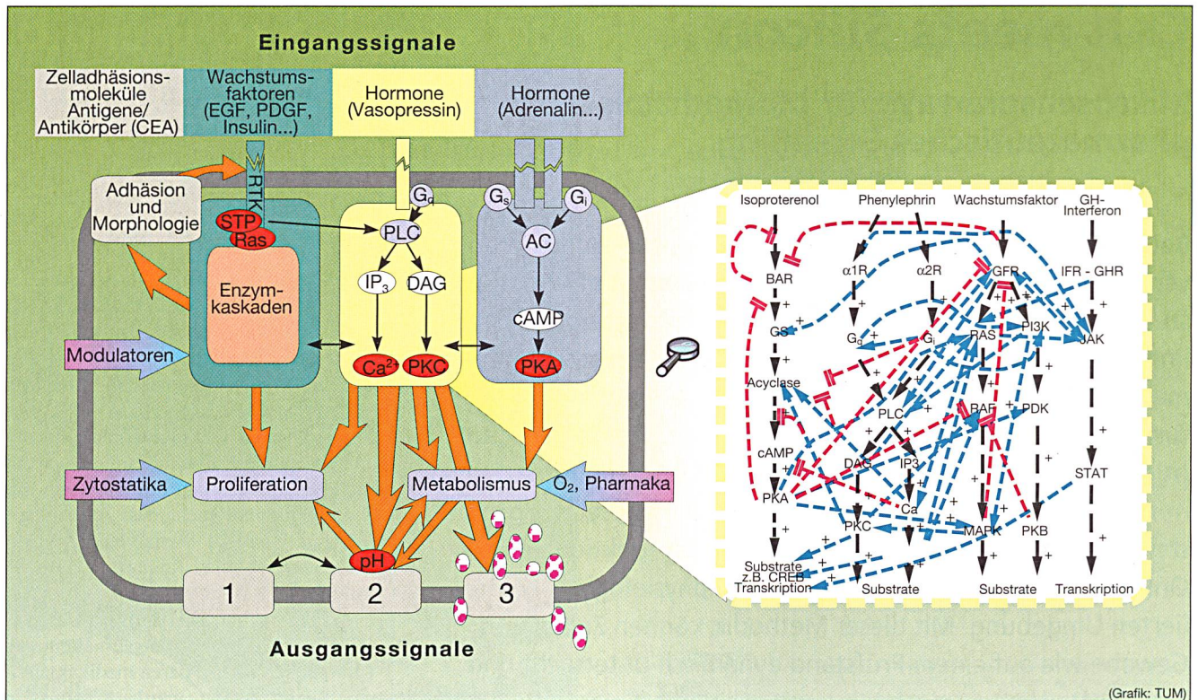
Bild 1 Schematische Darstellung der Komplexität interagierender Signalverarbeitungs- und Stoffwechselwege in der Zelle Die rechte Seite wurde aus [3] übernommen. 1: Membranpotenzial, Ionen (Na, K, Ca, Cl ...), dielektrische Eigenschaften der Zellmembrane; 2: pH der Mikroumgebung; 3: Metaboliten, Milchsäure, CO 2 , Reaktionswärme
