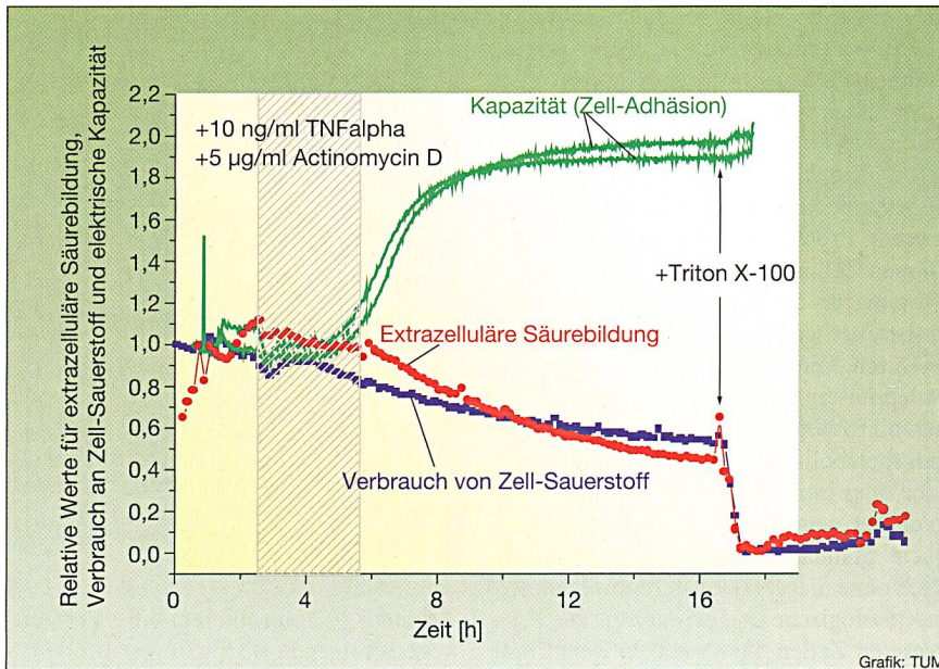
Bild 6 Messresultate einer Zellkultur auf Glas-Sensorchips
