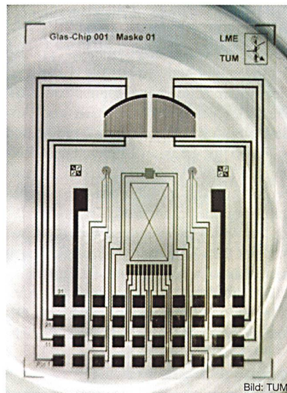
Bild 2 Glas-Sensorchip für mikrophysiologische Studien an zellulären Präparaten bei gleichzeitiger Lichtmikroskopie Der Chip enthält Sensorelemente für die Messung von Temperatur, pH-Wert, Sauerstoff und Impedanz. Durch geschickte Ankopplung eines Liquid-Handling-Systemes können Online-Informationen über Stoffwechselvorgänge und zellmorphologische Veränderungen gewonnen werden.
