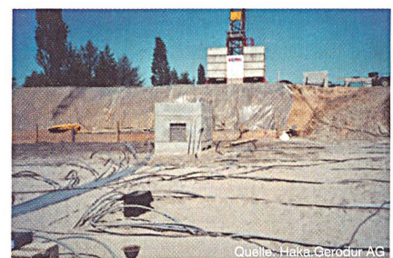
Bild 6 Ausbauarbeiten am Erdwärmespeicher in Neckarsulm-Amorbach
