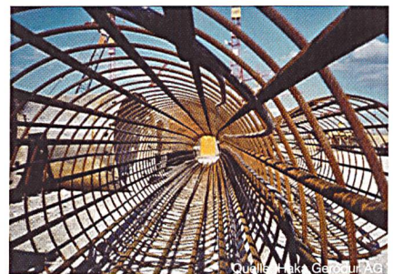
Bild 7 Energiepfahl für Unique Zurich Airport
