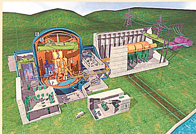
Réacteur nucléaire EPR/ Computerzeichnung des EPR (Bild Framatome ANP/ Siemens).
