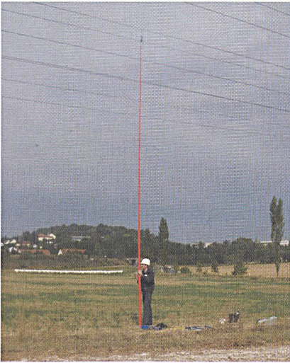
Modularer Spannungsprüfer von Dehn+Söhne
