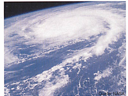
Eine der speziellsten Arten der Wolkenbildung. Im Bild: Hurricane Frances, aufgenommen am 27. August 2004 von der International Space Station (ISS), 230 Meilen über dem Sturm.
