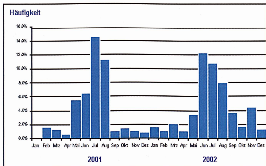
Häufigkeit der Störungereignisse pro Jahr auf der Höchstspannung 220 kV / 380 kV.
