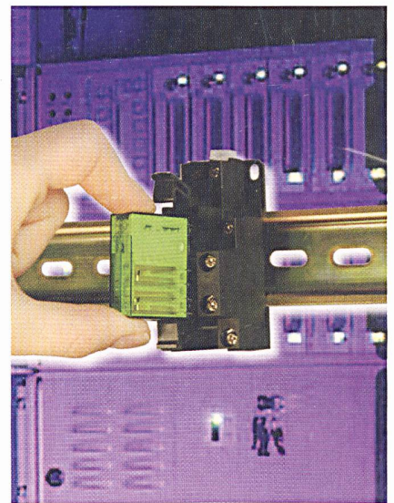
DIN-Schienen-Sockel SRD-SIM4 für Elesta-Sicherheitsrelais
