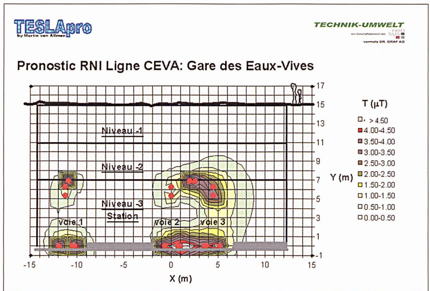
Bild 2 Querschnitt durch den unterirdischen Bahnhof Gare des Eaux-Vives mit Stromleitern und berechneten Linien gleicher magnetischer Flussdichte in Mikro-Tesla (Mittelwert über 24h-Fahrplanzyklus).
