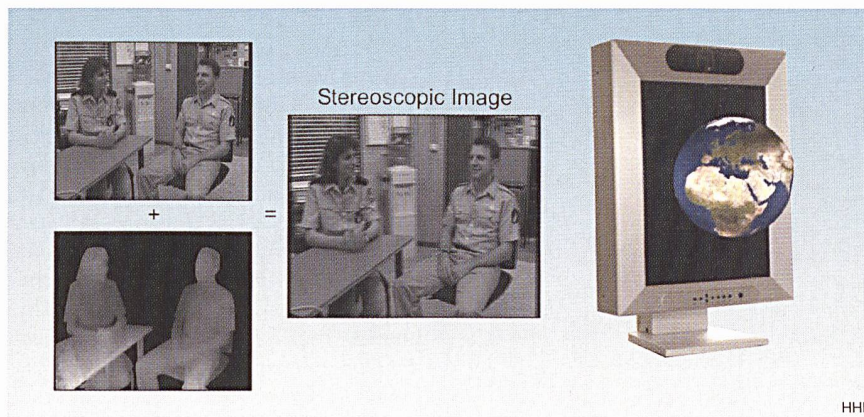
Bild 3 Erzeugung von Stereobildern aus einem Video und Tiefenkarte, autostereoskopisches Display
