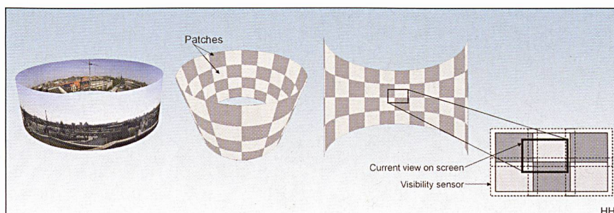
Bild 6 Effiziente Repräsentation von hochauflösendem Rundumvideo mit MPEG-4
