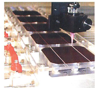
Solarzellenkonzepte: berührungslose Kontaktierung mit leitfähigen Kunststoffen.
