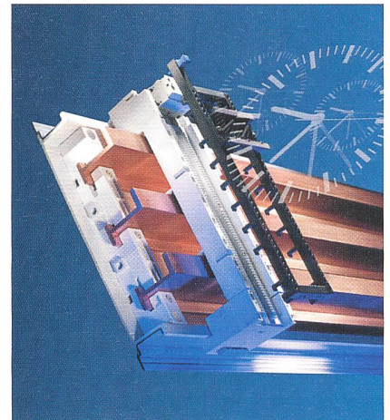
Sammelschienenhalter mit integrierter Querschnittanpassung
