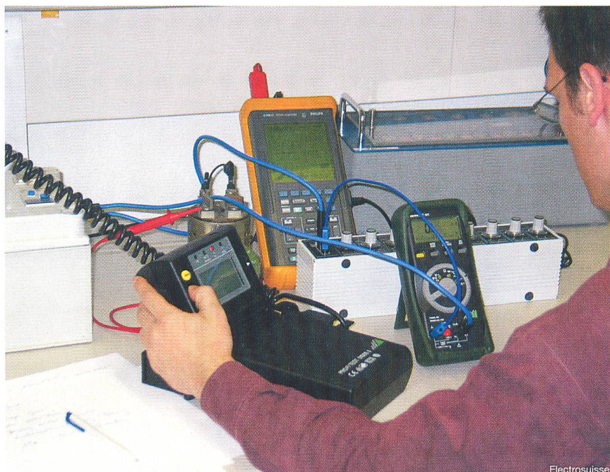
Bild 1 Eines der Geräte beim Test im Electrosuisse-Kalibrierlabor in Fehrlortorf
