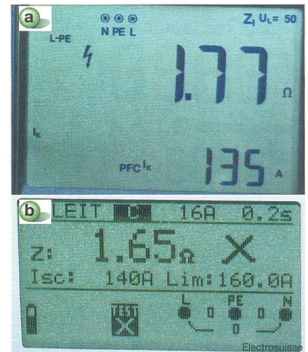
Bild 2 Unterschiedliche Displays
