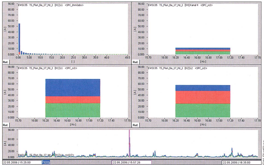
Bild 3 Wie sich der Bahnrückstrom in der Transformatorstation des EW Dietlikon verteilt 58 A (Mitte rechts) fließen in die Erdungsschirme der Mittelspannungskabel, der Rest von 12 A (im Bild oben rechts) in die Netz-PEN-Leiter der NS-Kabel
