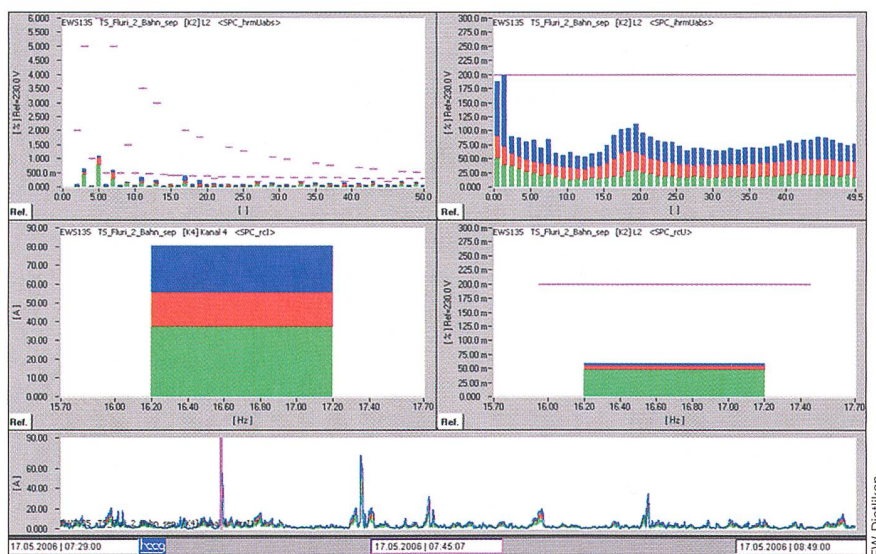
Bild 4 16,7-Hz-Anteil im EW-Netz
