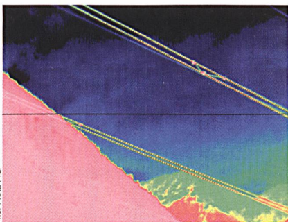
Bild 6 Thermovisionsbild des Leiterseils.
