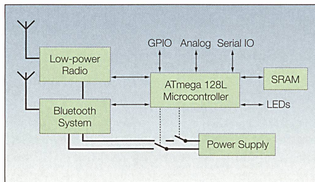
Figure 2 L'architecture du système BTnode rev3.
