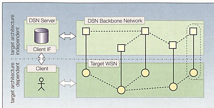
Figure 4 Architecture du réseau de support au déploiement.
