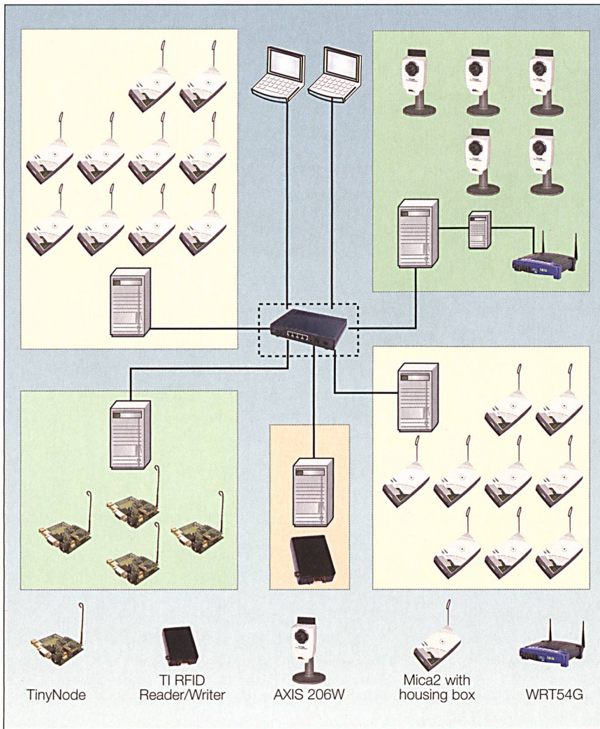
Figure 5 Une configuration des capteurs globaux (GSN) typique.
