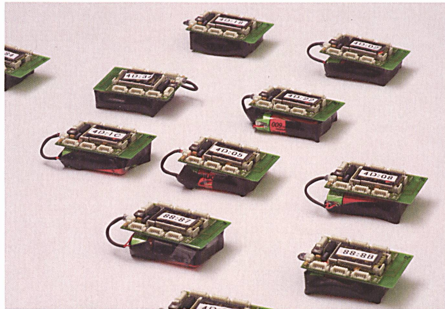
Figure 3 Les BTnodes développés à l'ETHZ.
