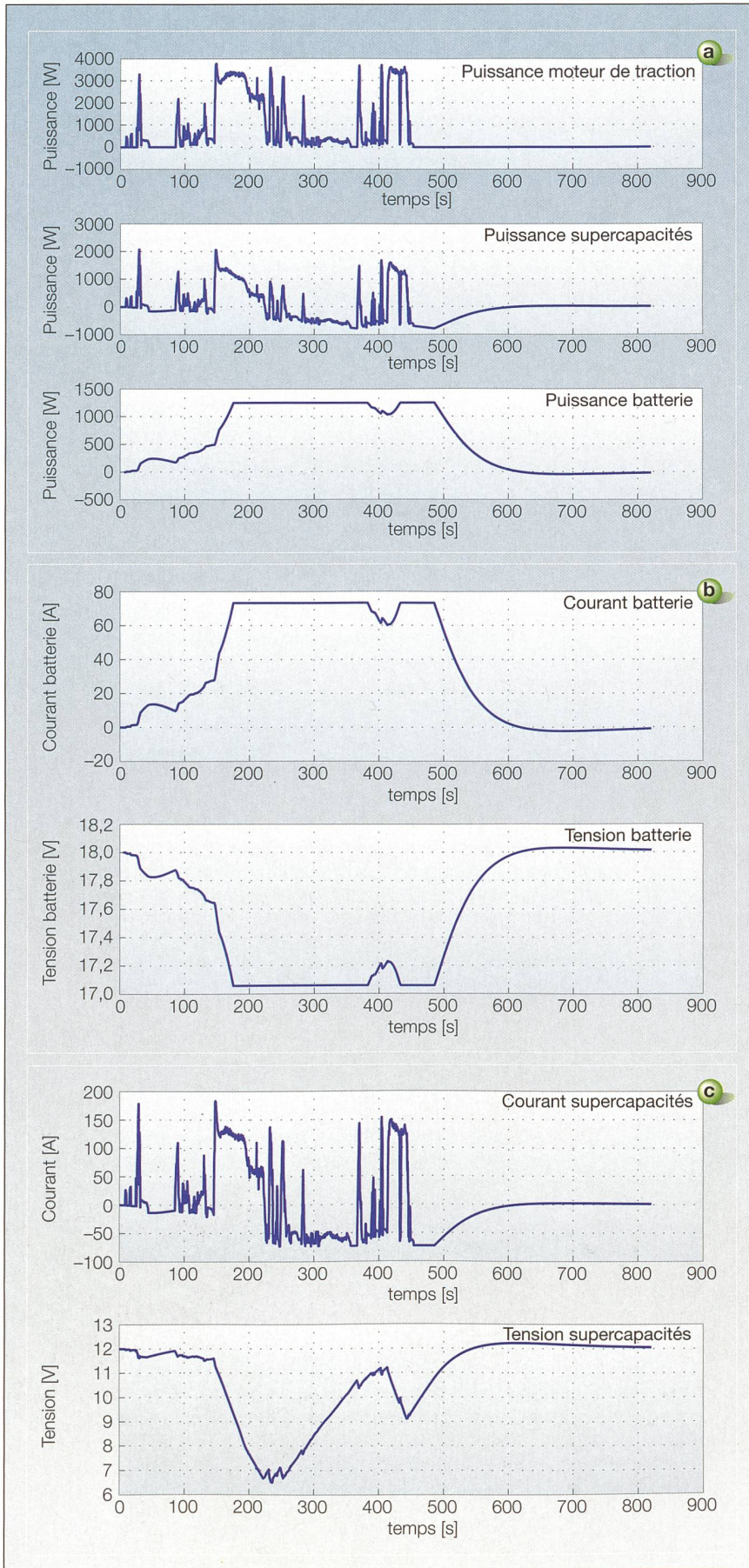
Figure 7 Courbes simulées des grandeurs électriques du système assisté en puissance. Figure 7a: puissances dans le véhicule; figure 7b: sollicitation de la batterie; figure 7c: sollicitation des supercondensateurs.
