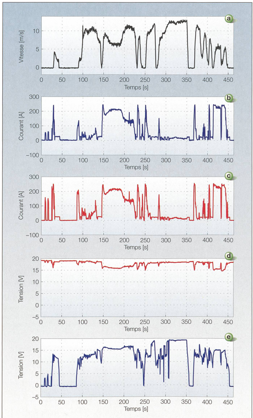
Figure 3 Courbes enregistrées sur un parcours type en ville de Lausanne. Figure 3a: Vitesse. Figure 3b: Courant batterie. Figure 3c: Courant moteur. Figure 3d: Tension batterie. Figure 3e: Tension moteur.
