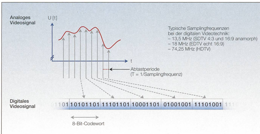
Bild 6 Umwandlung analog-digital.
