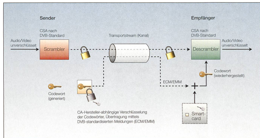
Bild 10 Verschlüsselte Übertragung.
