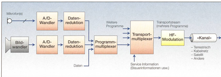
Bild 5 Digitale Fernsehübertragung.
