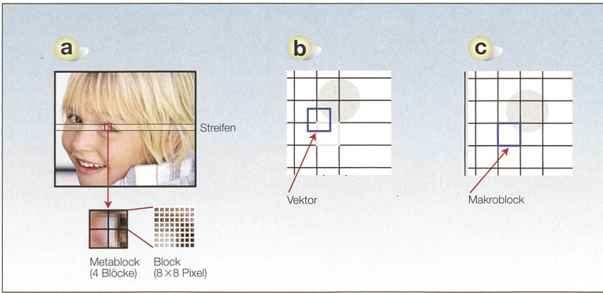
Bild 7 MPEG-Video-codierung.
