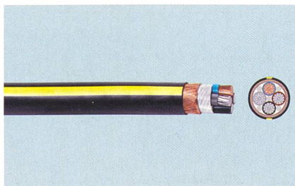
GKN-TNS-Kabel für den 5-Leiter-Hausanschluss mit Aluminium-Polleitern und einem Neutralleiter aus Kupfer.
