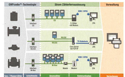
Topologien von GWF zur spartenübergreifenden Auslesung von Strom-, Gas- und Wasserzählern.
