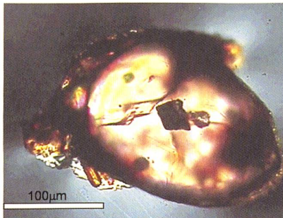
Ein Diamanteinschluss in einem Zirkon (Durchlichtaufnahme).
