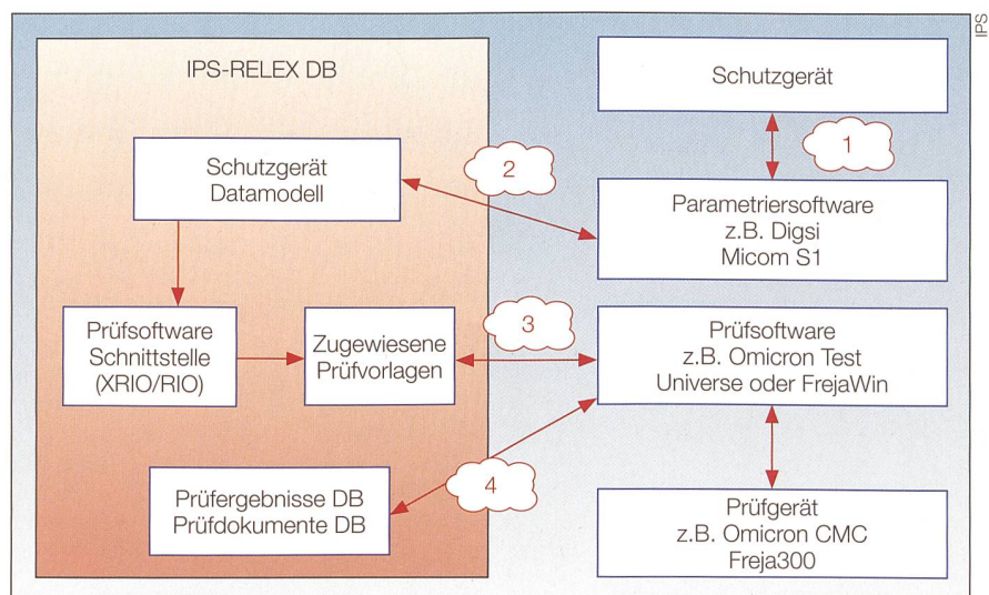
Bild 6 Prüfungsablauf.
